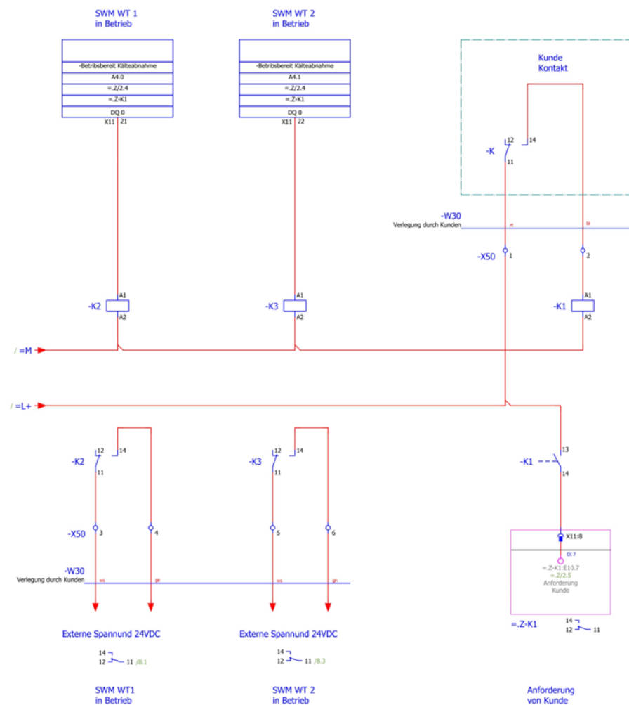
1.2 Muster - 2 Wärmetauscher
