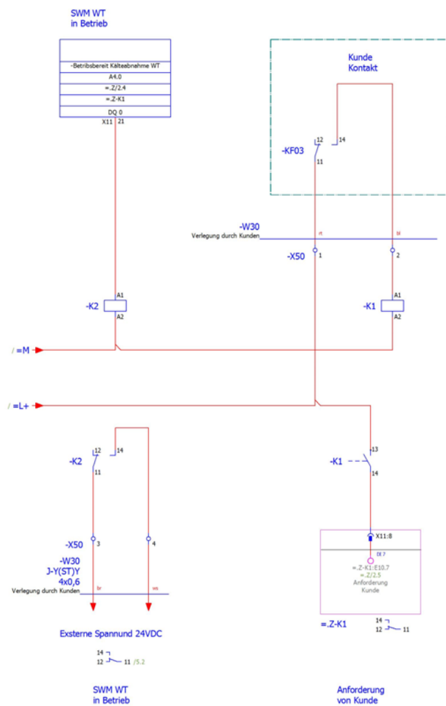
1.1 Muster - Wärmetauscher
