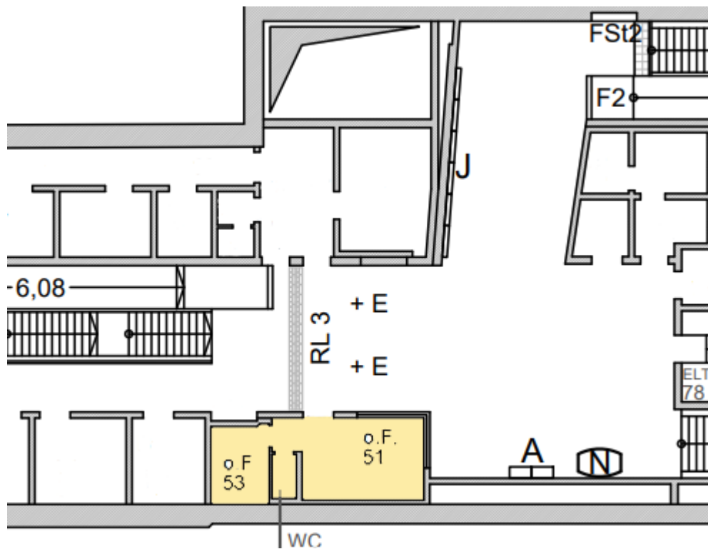
Lageplan
