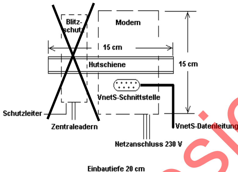
Abbildung 3: Modemeinbau
