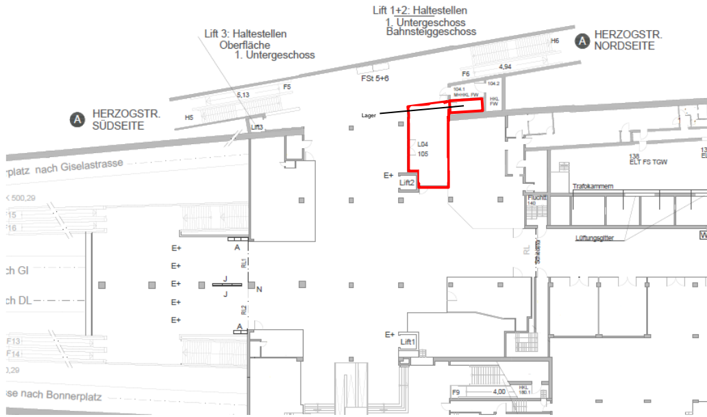
Lage ME 04 + Lager im Sperrengeschoss
